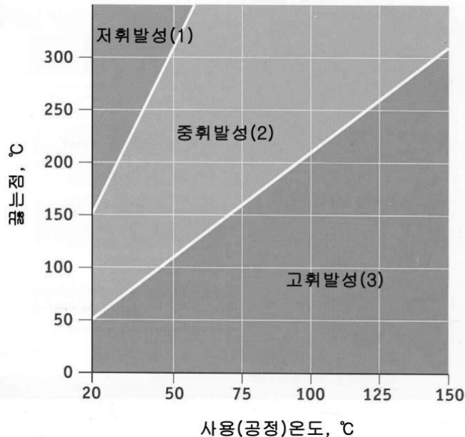
〈그림〉 끓는점과 사용(공정)온도에 따른 휘발성 분류그래프
