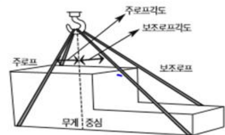
〈그림18〉 중심이 치우친 하물의 로프걸기
