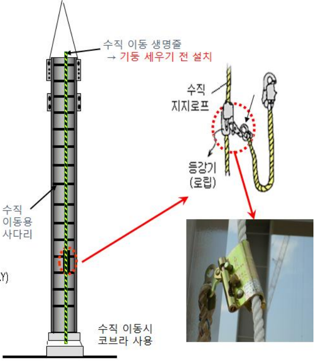
승강트랩, ROPE 고정점 상세도 SCALE: 1 / 10
