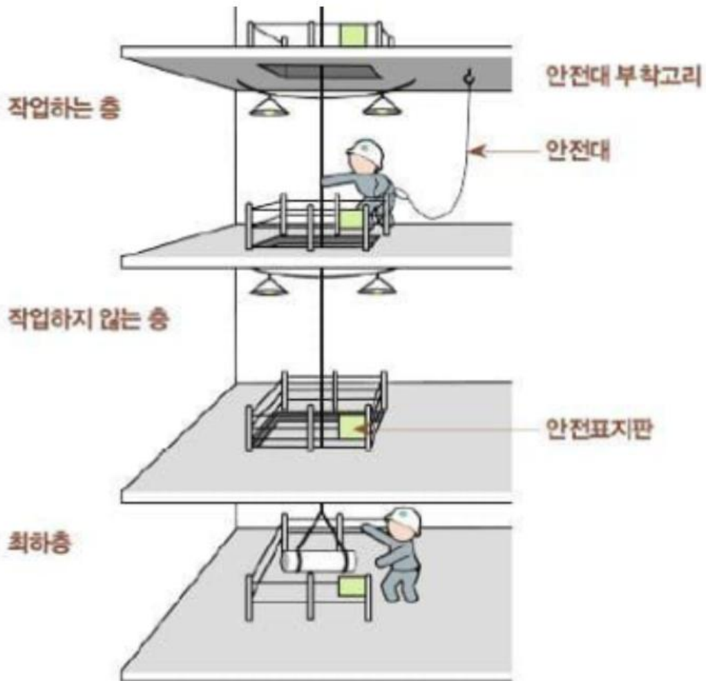
작업용 개구부의 방호조치 개념도
