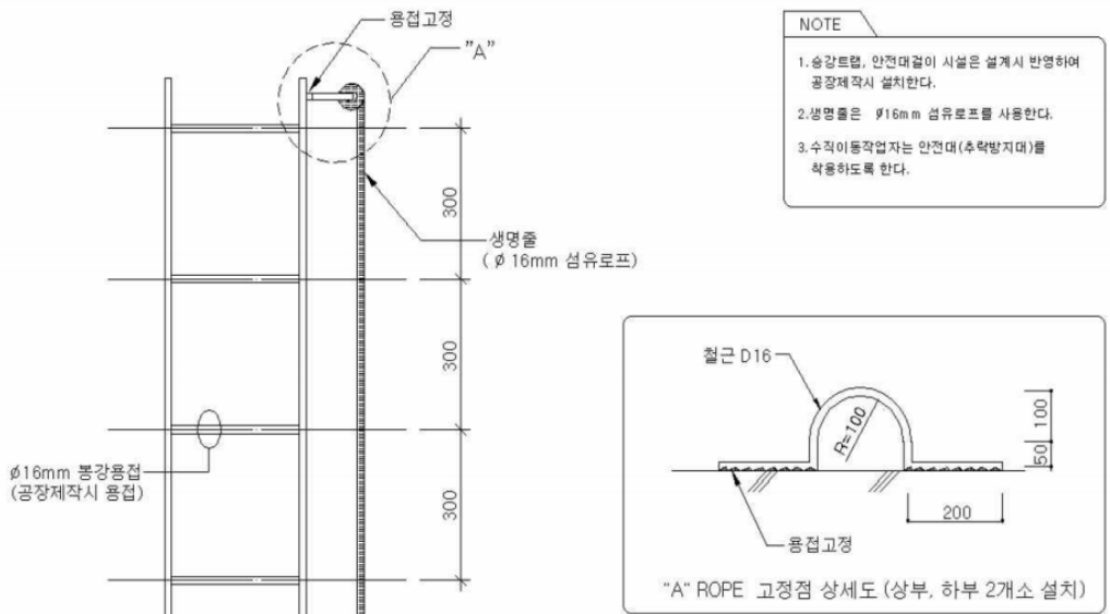
승강트랩, ROPE 고정점 상세도 SCALE: 1 / 10
