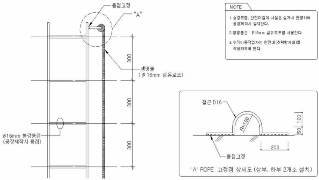
승강트랩, ROPE 고정점 상세도 SCALE: 1 / 10
