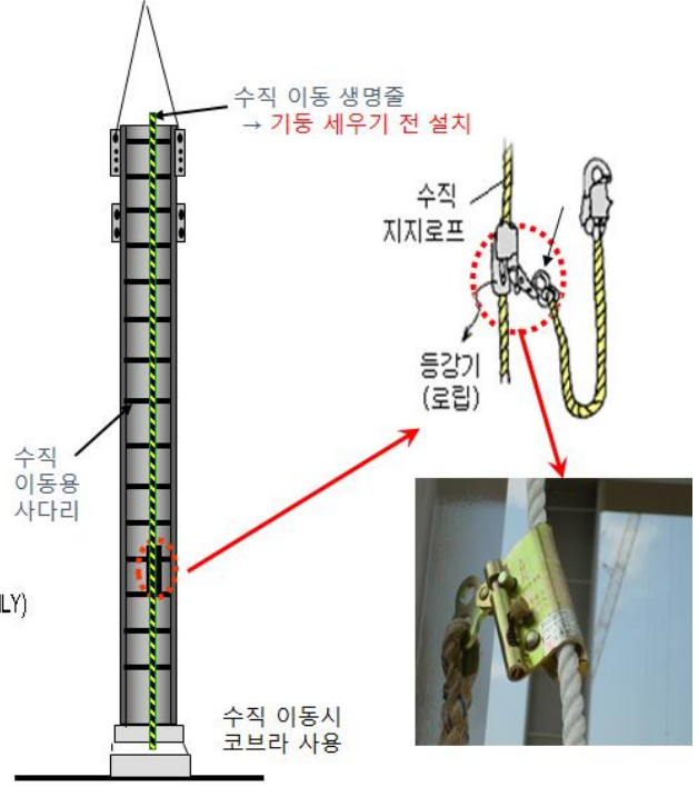
승강트랩, ROPE 고정점 상세도 SCALE: 1 / 10
